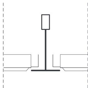
PARMA ENRASADA
