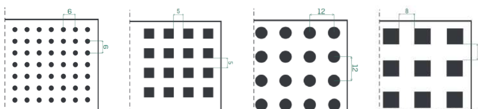
Perforado Ø2,5 U | 13% perforado M | 25% perforado ML | 6% perforado
