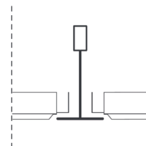
BANDEJA CAPRI ENRASADA (T-24)
