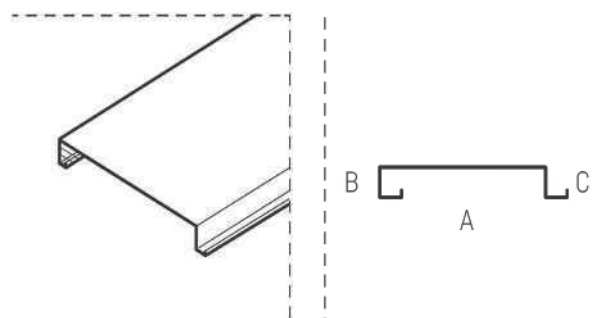
LAMA VENEZIA LISA
