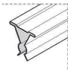
PERFIL OCULTO TRIÁNGULO
