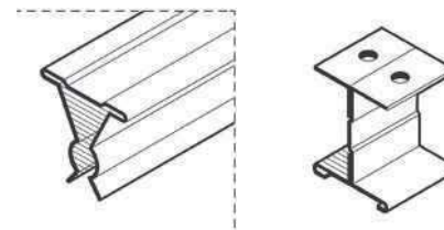
PERFIL OCULTO TRIÁNGULO
