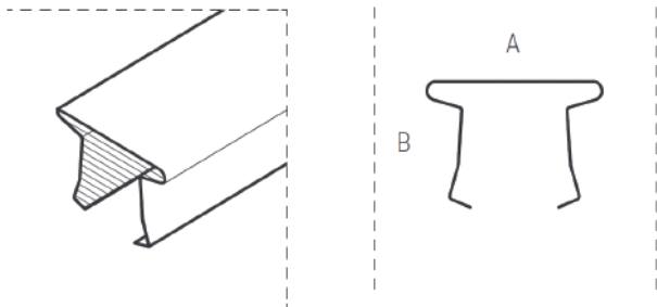
JUNQUILLO
