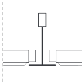
MÓDENA ENRASADA
