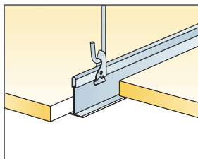
Suspensión con varilla y Clip de cuelgue
