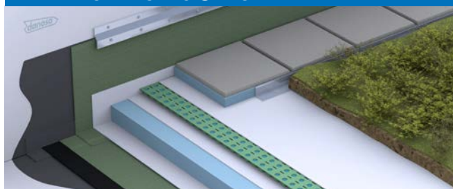
SISTEMA PRO8 GLASDAN® PRO 30 P | POLYDAN® PRO 50/GP GREEN GARDEN
