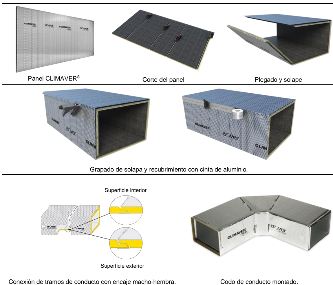
Figura A.1: Descripción general del montaje de segmentos de conducto.
