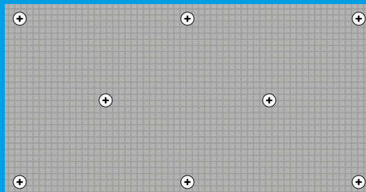
Fig.1 En paneles de 1200 x 600 mm usa 8 arandelas o pasadores o tacos de expansión.
