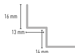
ALETA 10 Galvanizado ALETA 11 Prelacado Blanco
