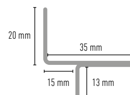
ALETA 9 Prelacado Blanco
