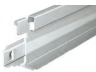
2: Perfil secundario Chicago Metallic T24 Click 2890 (-2894)
