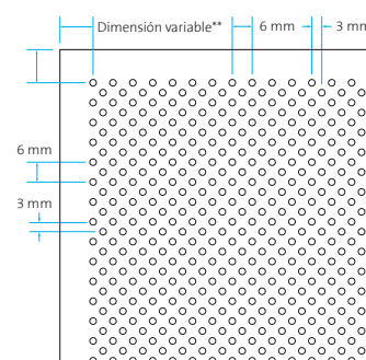
Perforación Ø 2 mm Área perforada ~ 18%
