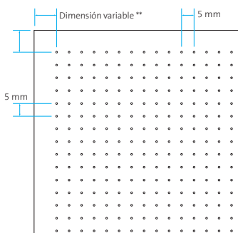
Perforación ultra-micro Ø 0,7 mm Área perforada ~ 1,5%
